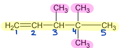
3,4,4-trimethyl-1-pentene
