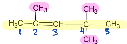
2,4,4-trimethyl-2-pentene
